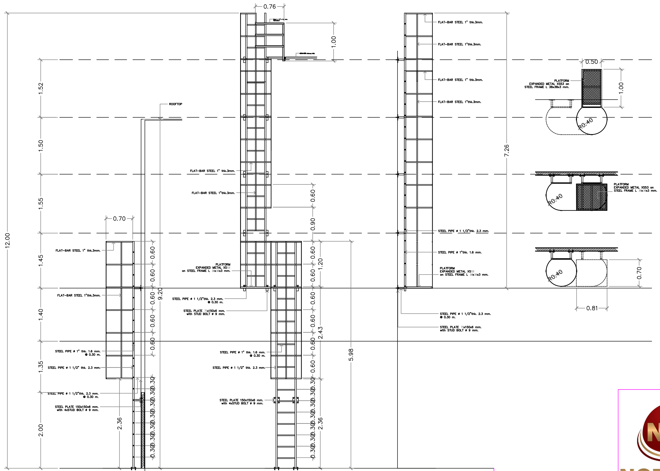
แบบขยายการติดตั้งบันได 2 = 1SET มาตราส่วน 1 : 50
